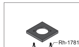
Sh-1506 Chapetón con Tornillos Screws with Escutcheon
